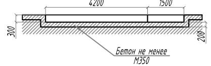
Разрез А -А
